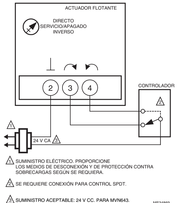
Fig. 6. MN6105 con control On/Off (encendido/apagado).
