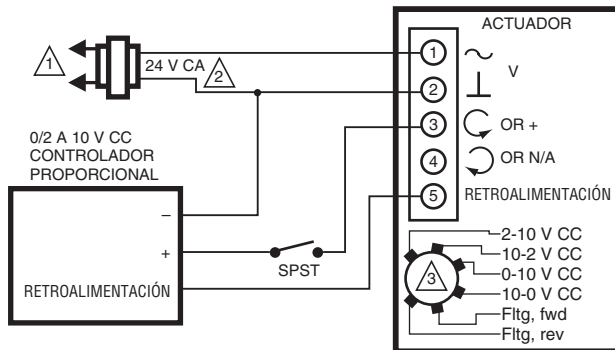
Fig. 17. MS7505 con control de sobrecomando para la posición completamente abierta (configuración del modo de modulación).
