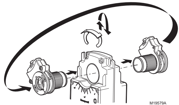
Fig. 23. Montage de l'accouplement de l'arbre sur le côté opposé de l'actionneur.
