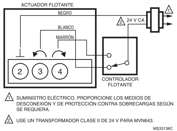
Fig. 11. MVN613 o MVN643 con control de dos posiciones.
