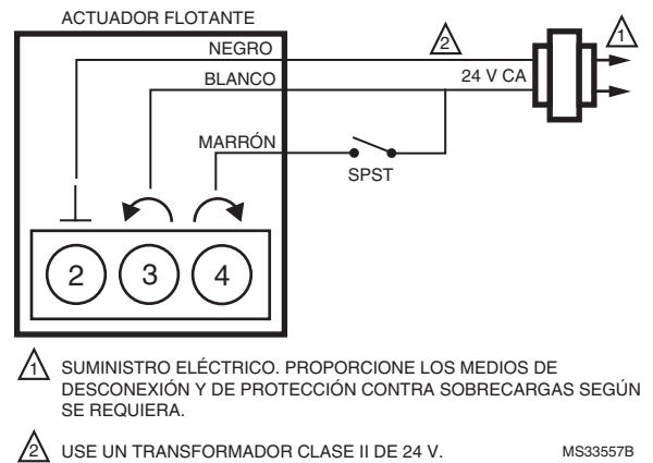
Fig. 12. MVN643 con control SPST de dos posiciones.
