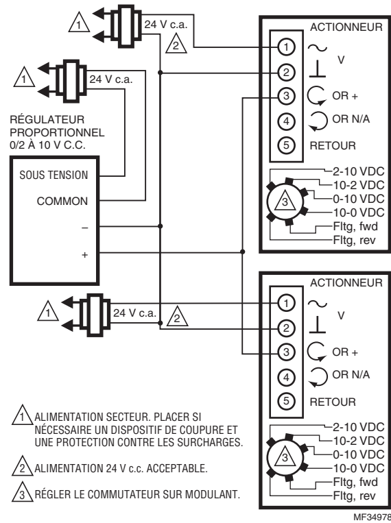
Fig. 22. MS7505 avec régulateurs proportionnels actionnant plusieurs actionneurs (réglage en mode modulant).
