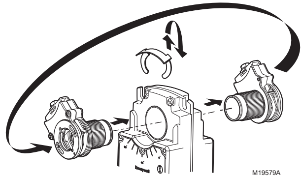
Fig. 23. Colocación del acoplador del eje al actuador en el lado opuesto.
