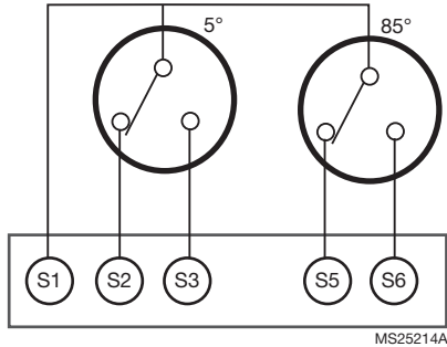
Fig. 9. Cableado para el modelo con interruptores aux./terminales.
