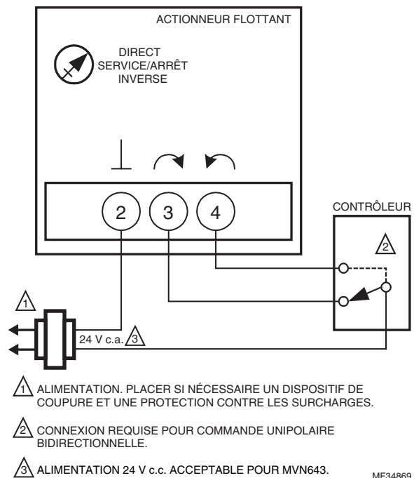
Fig. 6. MN6105 pour action Marche/Arrêt.
