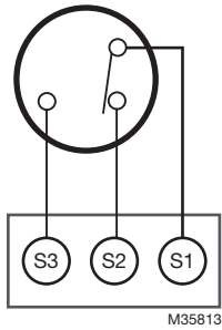
Fig. 21. Câblage pour les modèles avec interrupteurs d'extrémité/auxiliaire.
