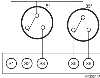
Fig. 9. Câblage pour les modèles avec interrupteurs d'extrémité/auxiliaire.
