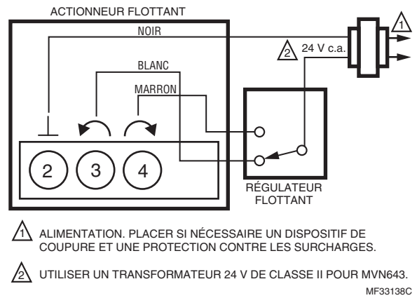
Fig. 11. MVN613 ou MVN643 avec commande à deux positions.
