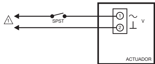
Fig. 19. MS7505 con controles proporcionales (configuración del modo modulante).
