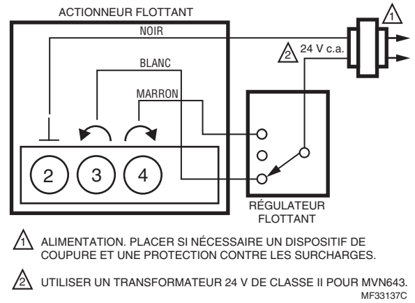
Fig. 10. MVN613 ou MVN643 avec commande flottante
