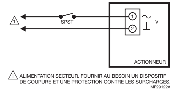
Fig. 20. MS4105 commande à deux positions de tension secteur (120 V).
