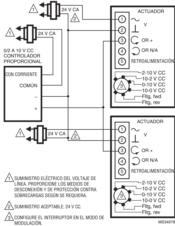
Fig. 22. MS7505 con controladores proporcionales que hacen funcionar múltiples actuadores (configuración del modo de modulación).
