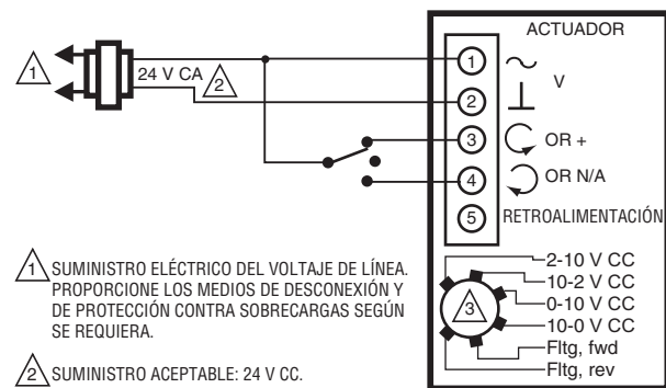
Fig. 16. MS7505 con control flotante (configuración del modo flotante).
