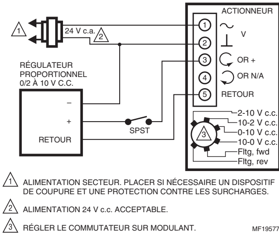
Fig. 18. MS7505 avec dérivation pour fermeture complète (réglage en mode modulant).
