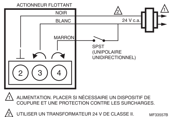
Fig. 12. MVN643 avec commande unipolaire unidirectionnelle à deux positions.
