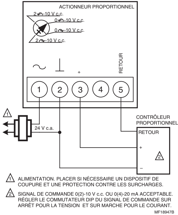
Fig. 8. MN7505 pour action modulante.
