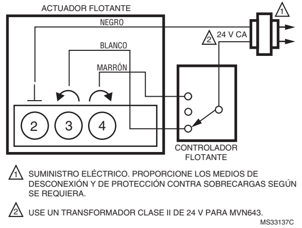
Fig. 10. MVN613 o MVN643 con control flotante.
