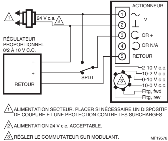
Fig. 17. MS7505 avec dérivation pour ouverture complète (réglage en mode modulant).
