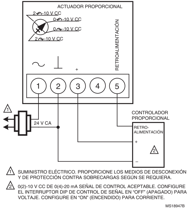
Fig. 8. MN7505 con control de modulación.
