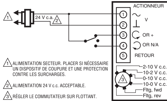
Fig. 16. MS7505 pour action flottante (réglage en mode flottant)
