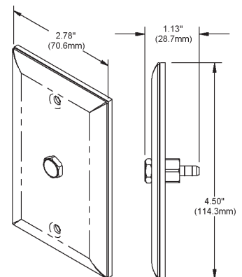
Fig. 9: Wall Plate (ZPS-ACC01)
