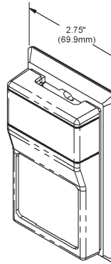
Fig. 8: Delta Style Enclosure (ZPS-ACC03)
