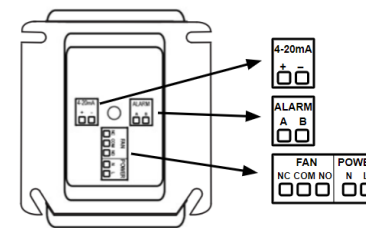
Figure 4 Vue arrière et connecteurs du détecteur de tension de ligne (Série 12)
