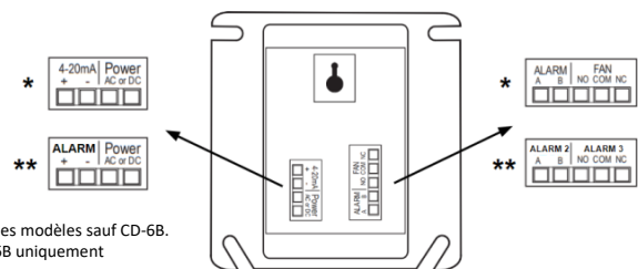
Figure 3 Vue arrière et connecteurs du détecteur basse tension (Série 6)
